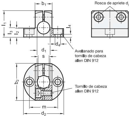
Kit de sujeción GN 511
